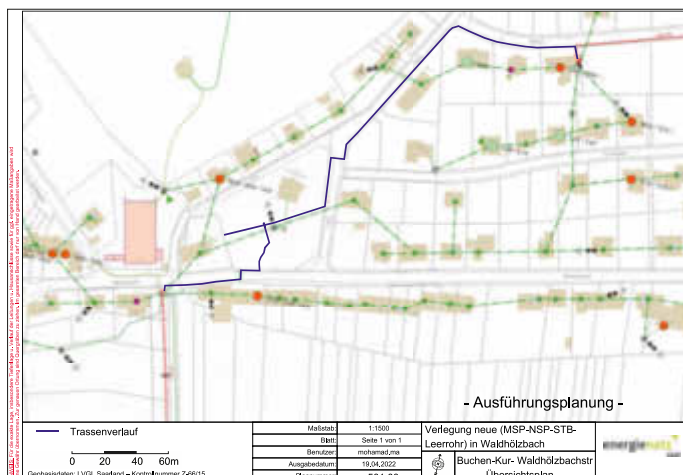
Ausführungsplanung - Trassenverlauf - Übersichtsplan
