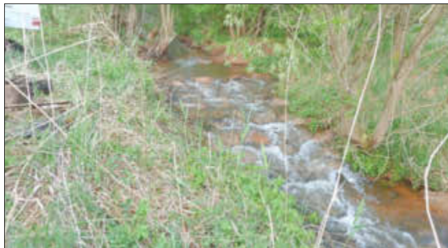
Nach dem Rückbau überwindet eine Raurampe den Höhenunterschied. Sie ist durch die Lücken zwischen den Steinen für alle Fische durchwanderbar.
